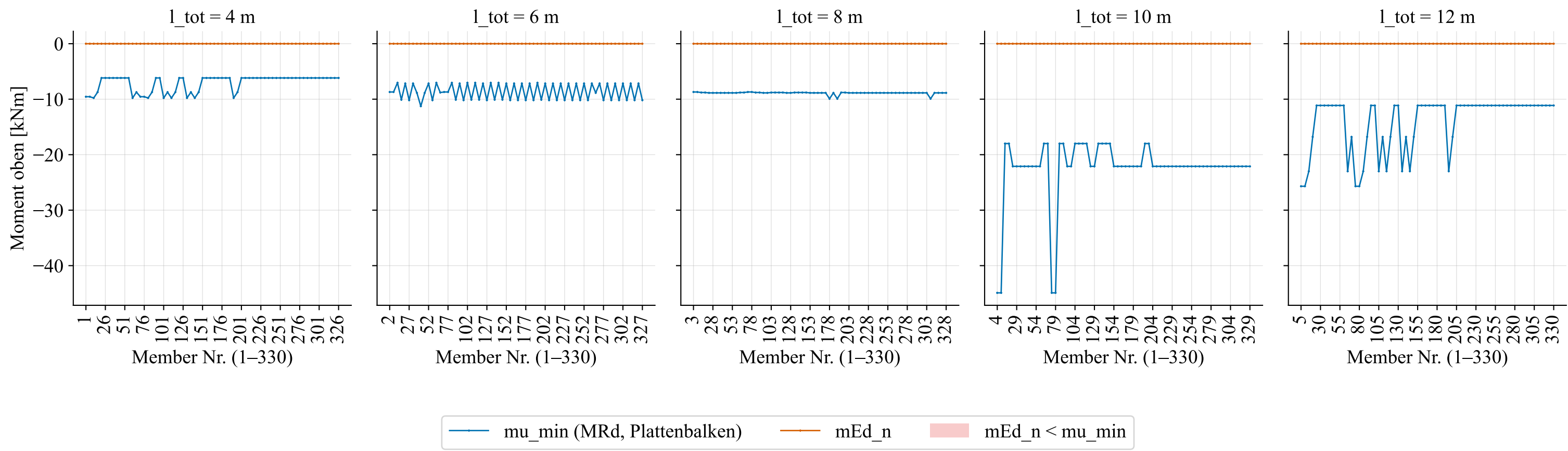
Biegewiderstand \mu_{\min} (MRd, Plattenbalken) vs. Bemessungsmoment mEd_n je Member, kategorisiert nach Spannweite (Members_rc_rib_simple_V3)
